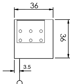
Profil du carter 36x36 entre 7m et 8m de base Alimentation à droite
